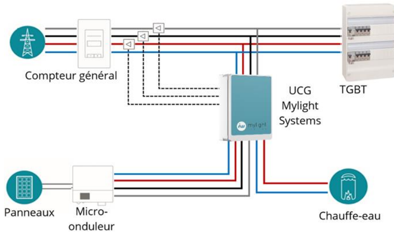
Figure 7. Cas d'utilisation typique et mise en armoire UCG-E9301-31-FR
