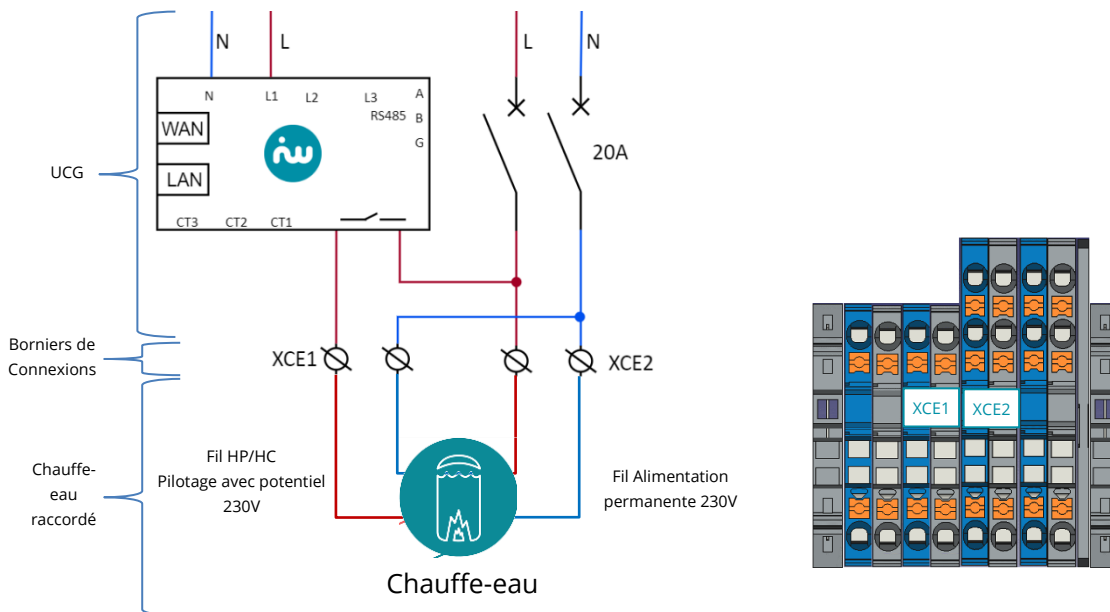
Figure 22. Schéma de pilotage d'un chauffe-eau monophasé avec un câble de puissance et de pilotage
