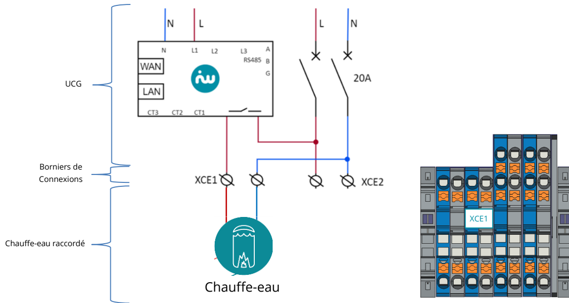
Figure 21. Schéma de pilotage d'un chauffe-eau monophasé avec un câble de puissance
