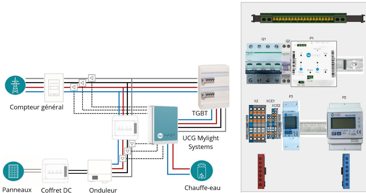
Figure 10. Cas d'utilisation typique et mise en armoire UCG-X0302-31-FR
