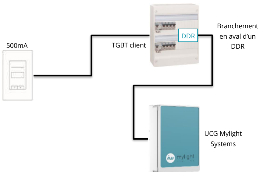
Figure 16. Schéma de raccordement unifilaire de l'alimentation pour les coffrets X
