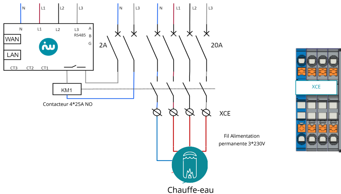
Figure 23. Schéma de pilotage d'un chauffe-eau triphasé avec un câble de puissance
