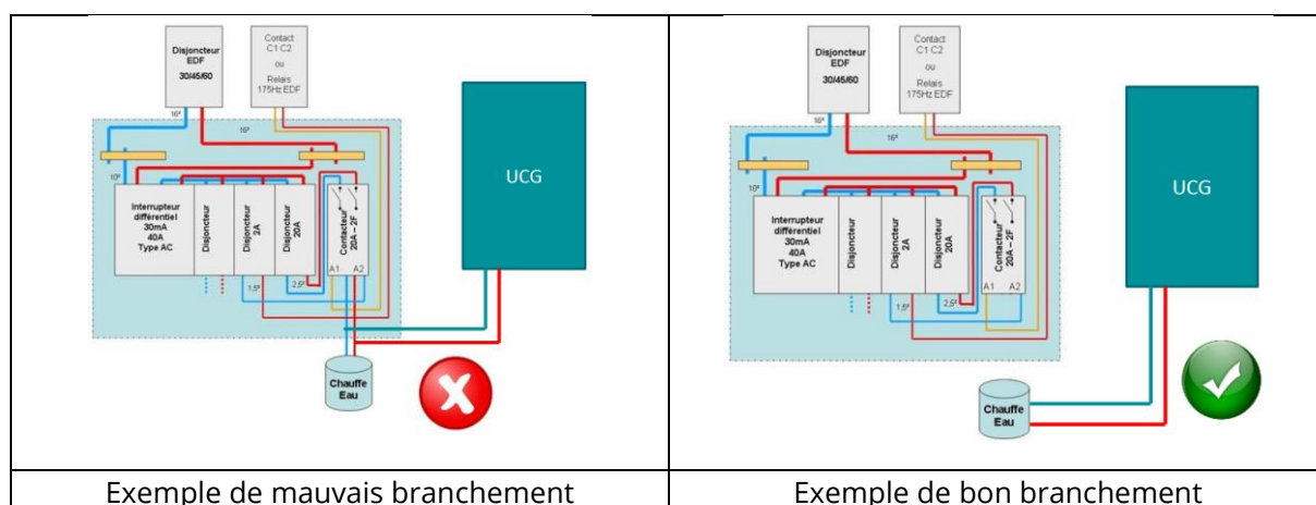
Figure 20. Principe de raccordement du chauffe-eau dans l'UCG
