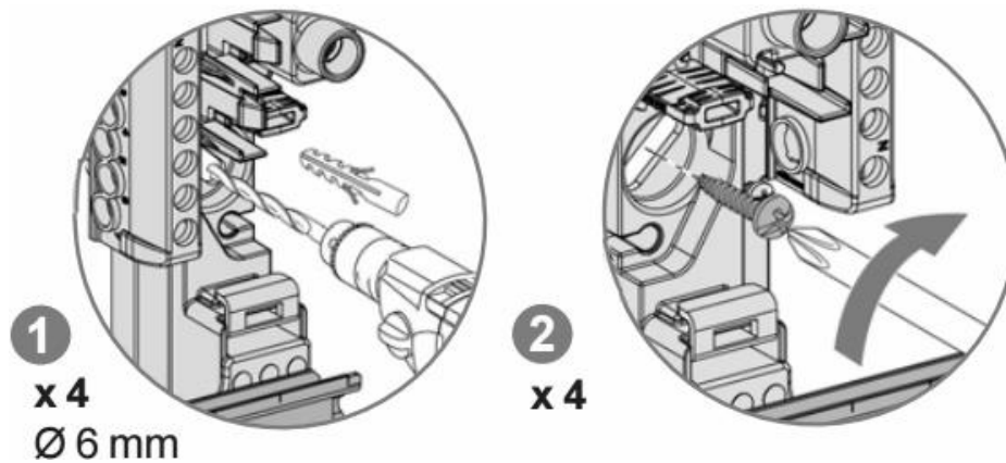
Figure 12. Montage de l'UCG sur un mur
