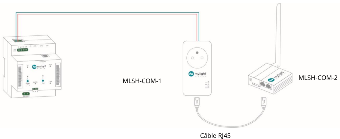
Figure 30. Connexion internet via le modem cellulaire et prise CPL
