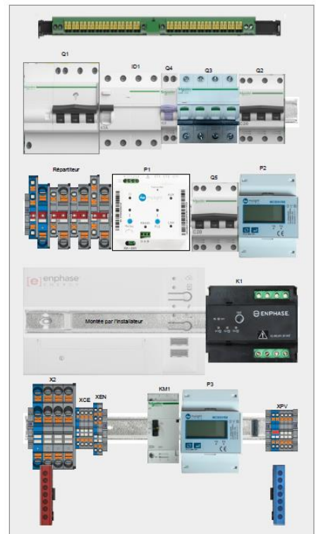
Figure 8. Cas d'utilisation typique et mise en armoire UCG-E9302-33-FR
