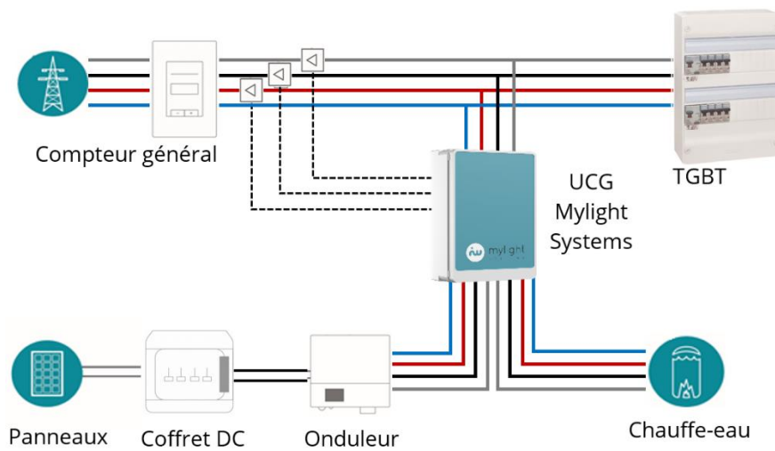
Figure 4. Cas d'utilisation typique et mise en armoire UCG-99302-33-FR
