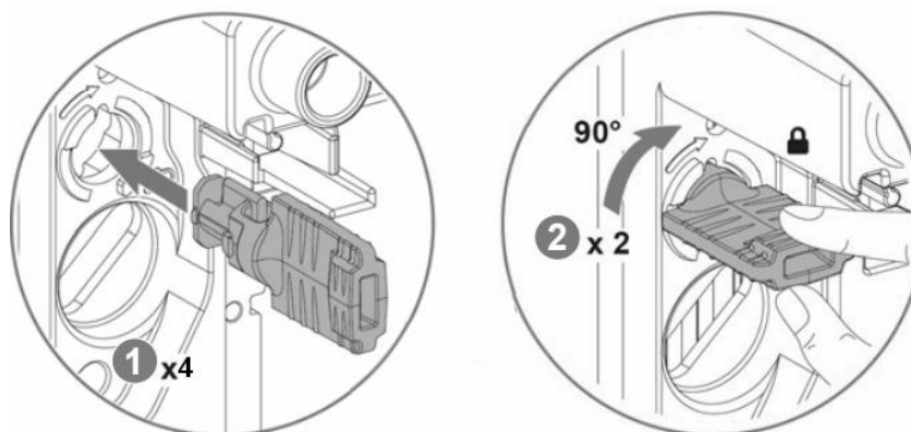
Figure 13. Montage de l'UCG sur gaines techniques
