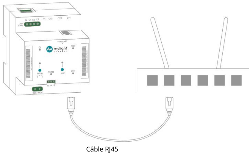
Figure 31. Schéma de connexion filaire entre MG3 et Box internet
