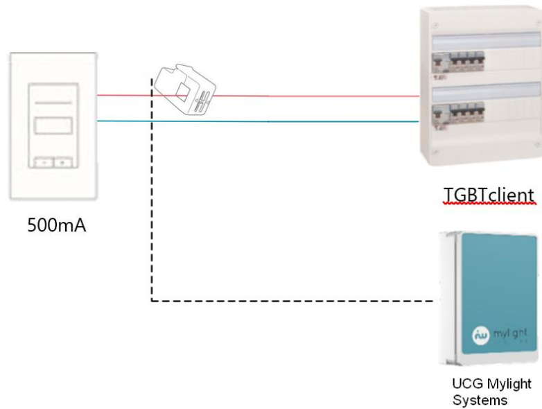
Figure 24. Schéma de placement des TC pour une alimentation monophasée sur le TGBT
