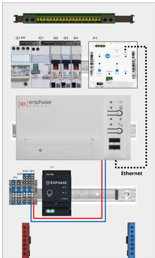
Figure 27. Schéma de principe de montage de la passerelle Envoy
