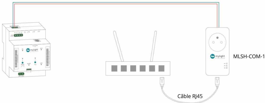
Figure 32. Schéma de connexion internet via la prise CPL
