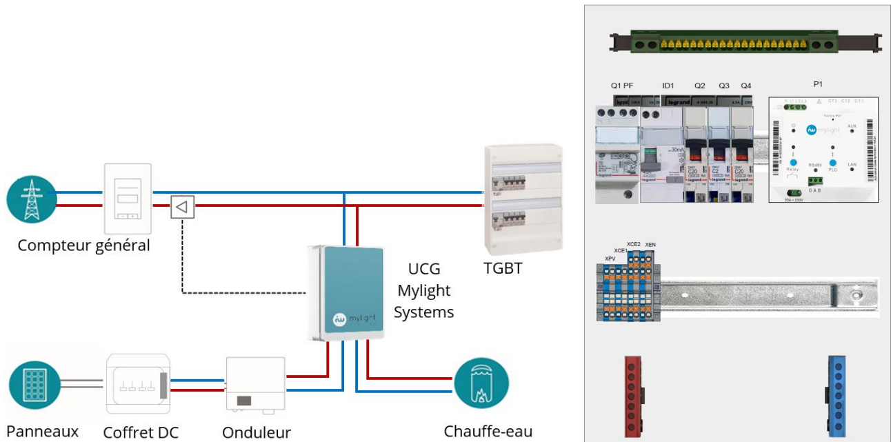
Figure 1. Cas d'utilisation typique et mise en armoire UCG-U4301-11-FR et UCG-U6301-11-FR
