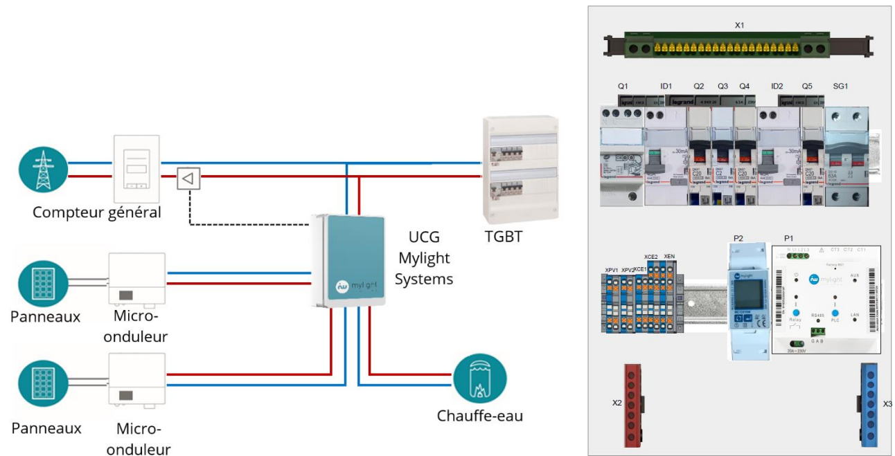
Figure 2. Cas d'utilisation typique et mise en armoire UCG-U8301-11-FR
