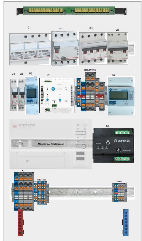
Figure 7. Cas d'utilisation typique et mise en armoire UCG-E9301-31-FR
