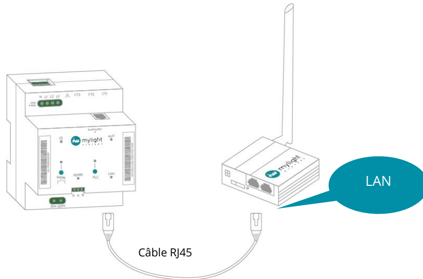
Figure 29. Schéma de connexion entre la MG3 et le modem cellulaire
