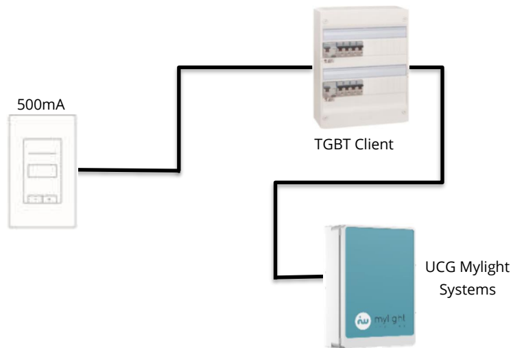
Figure 14. Schéma de raccordement unifilaire de l'alimentation sur le TGBT
