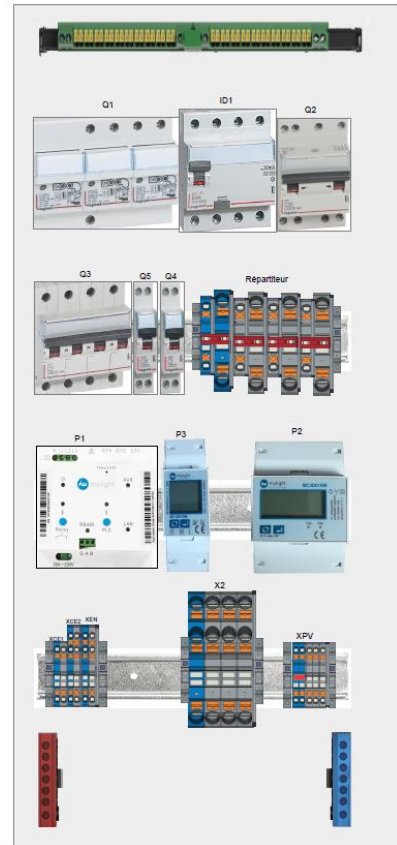
Figure 3. Cas d'utilisation typique et mise en armoire UCG-99301-11-FR
