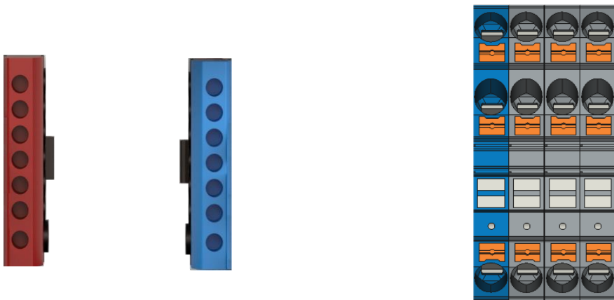
Figure 17. Borniers d'alimentation monophasé (gauche) et triphasé (droite)
