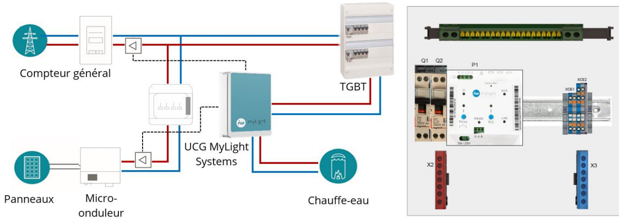
Figure 9. Cas d'utilisation typique et mise en armoire UCG-X0301-11-FR
