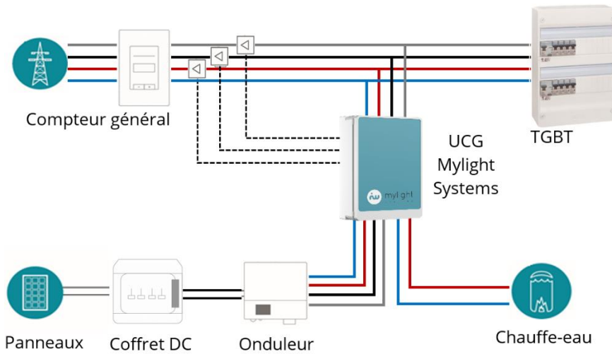
Figure 3. Cas d'utilisation typique et mise en armoire UCG-99301-11-FR
