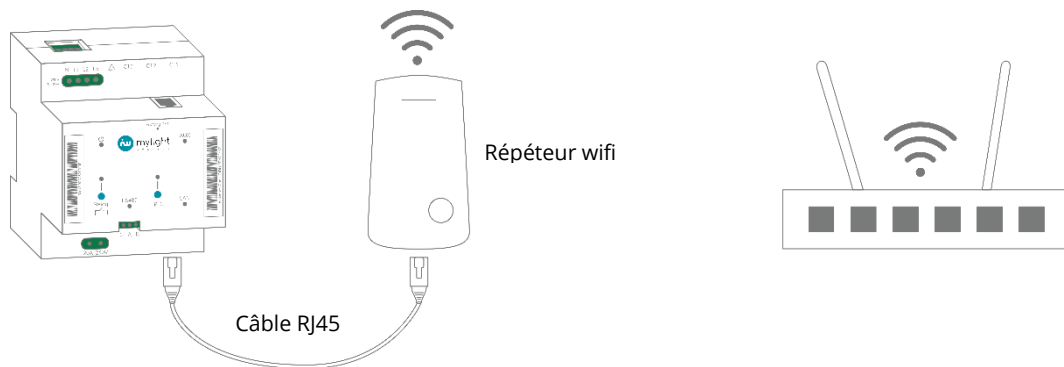
Figure 33. Schéma de connexion internet via répéteur wifi et box internet
