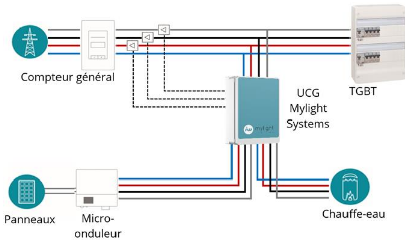
Figure 8. Cas d'utilisation typique et mise en armoire UCG-E9302-33-FR
