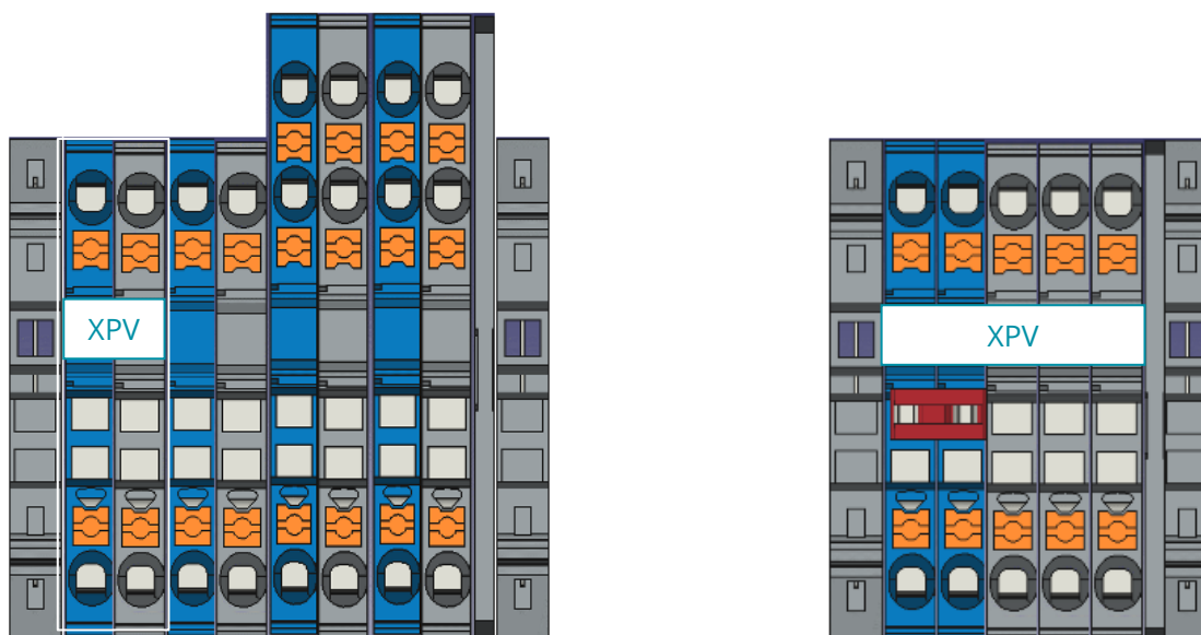
Figure 19. Borniers PV monophasés (gauche) et triphasés (droite)
