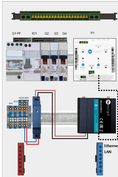
Figure 28. Schéma d'alimentation du modem via un convertisseur AC/DC sur rail DIN
