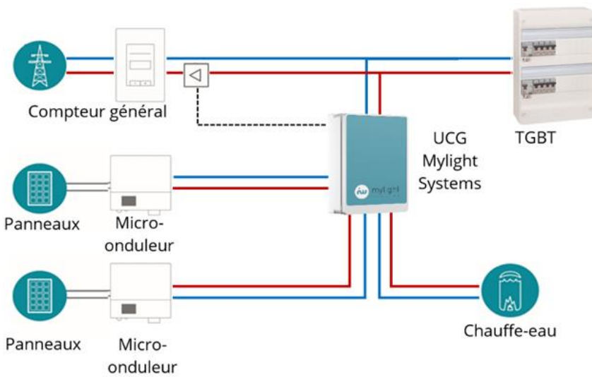
Figure 6. Cas d'utilisation typique et mise en armoire UCG-E8301-11-FR
